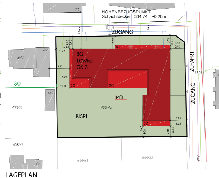
LAGEPLAN
